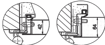
Neu Stahltür dw 42 und dw 64
