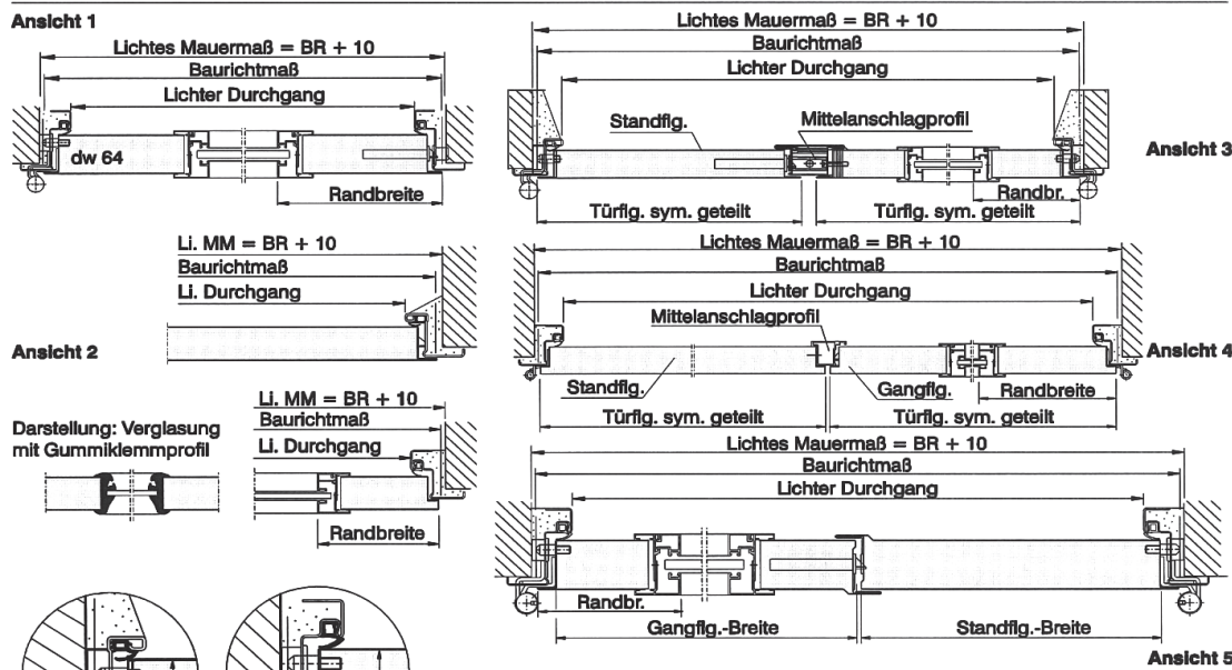
Neu Stahltür dw 42 und dw 64
